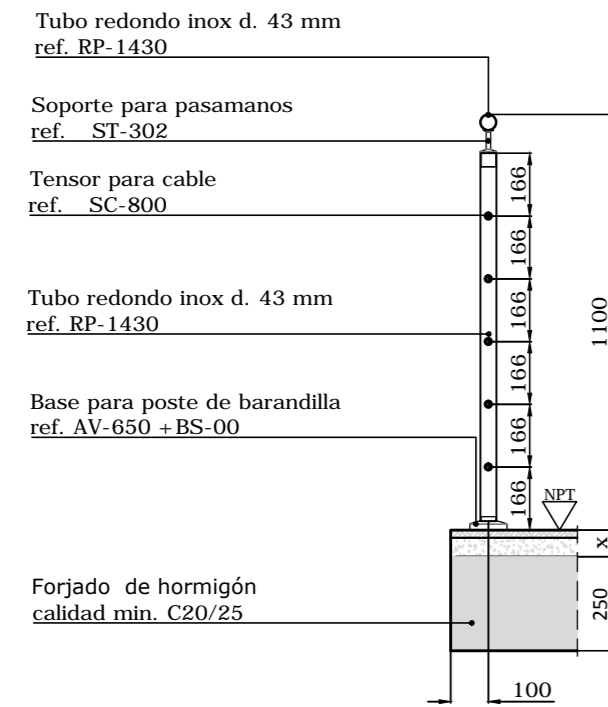
Sección A-A Barandilla R-Concept Easy Cable Montaje Superior AV-650 + BS-00 Escala 1:20
